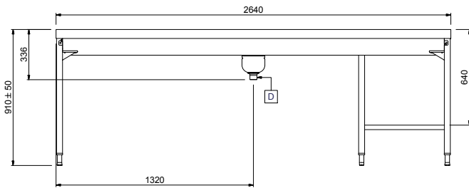
Front aanzicht
